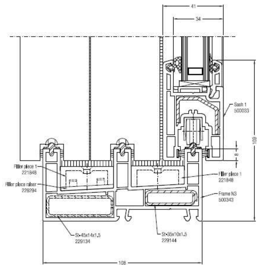
Sezione nodo 3 ante scorrevoli finestra
