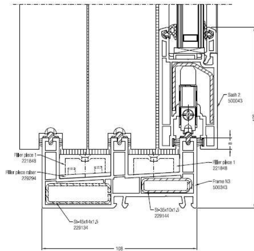
Sezione nodo 3 ante scorrevoli porta finestra
